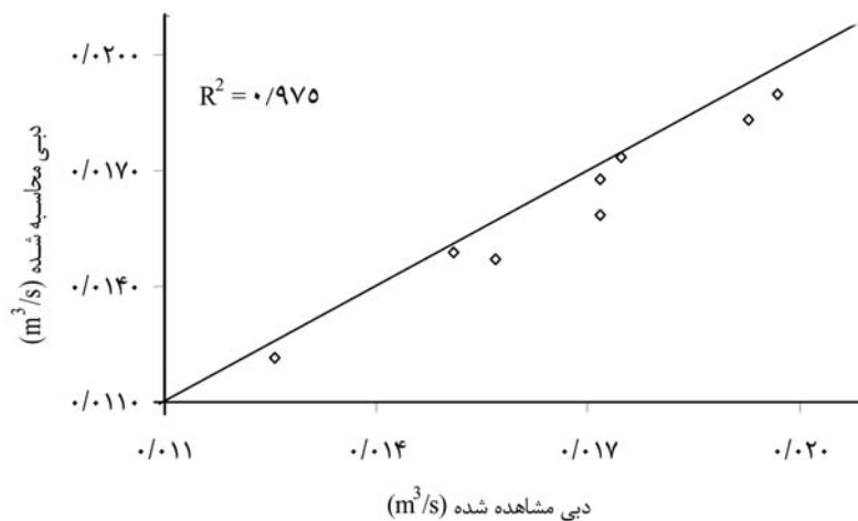
شکل ۱۴- تغییرات دبی محاسبه شده بر حسب دبی مشاهداتی ( \theta=115 درجه).
