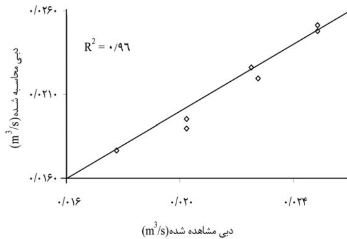
شکل ۱۳- تغییرات دبی محاسبه شده بر حسب دبی مشاهداتی ( \theta=90 درجه).
