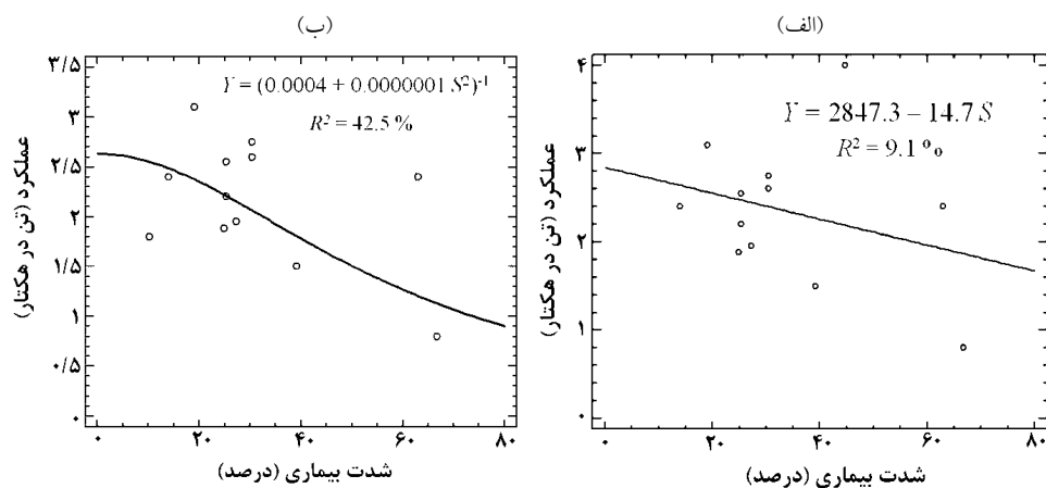
شکل ۱- رابطه رگرسیونی بین عملکرد محصول کلزا و شدت نهایی بیماری پوسیدگی اسکلویتینیایی ساقه به صورت دو مدل خطی (الف) و معکوس Y-X (ب).
