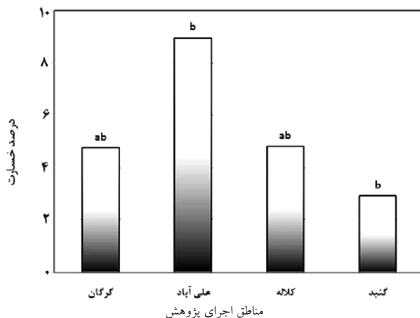
شکل ۳- درصد خسارت ناشی از بیماری پوسیدگی اسکروتینیایی ساقه در ۴ منطقه اجرای پژوهش در استان گلستان طی دو سال زراعی ۸۵-۸۶ و ۸۴-۸۵.
