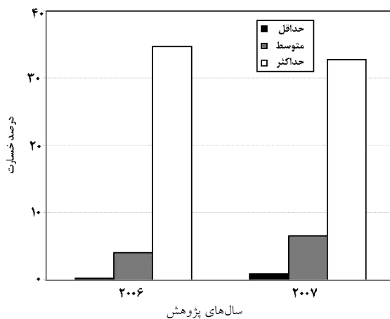
شکل ۴- درصد خسارت ناشی از بیماری پوسیدگی اسکروتینیایی ساقه در دو سال زراعی ۸۵-۸۶ (۲۰۰۶ میلادی) و ۸۶-۸۵ (۲۰۰۷ میلادی) در استان گلستان.
