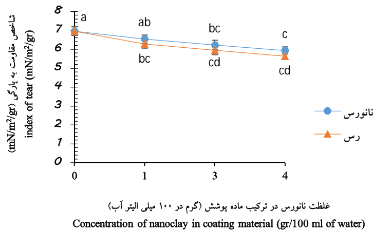
شکل ۷- تغییرات میزان شاخص پارگی در نتیجه مصرف مقادیر مختلف رس و نانورس به عنوان یک عامل پوششی در کاغذ. Figure 7. Changes rate of the of tear index as a result of different amounts consumption of clay and nanoclay as a coating on paper.
