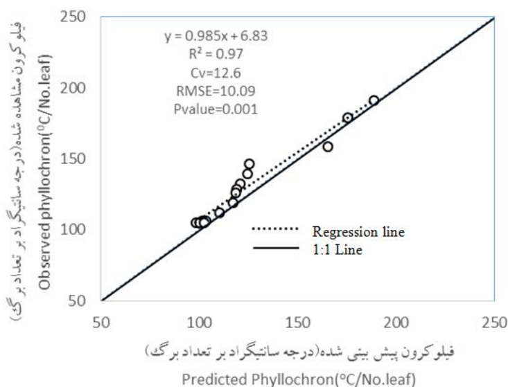
شکل ۳- برازش فیلوکرون مشاهده شده در برابر فیلوکرون پیش‌بینی شده در شرایط مطلوب توسط مدل.
