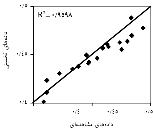
شکل ۲- ضریب دبی مشاهده‌ای و تخمینی در سرریز جانبی تخت.
