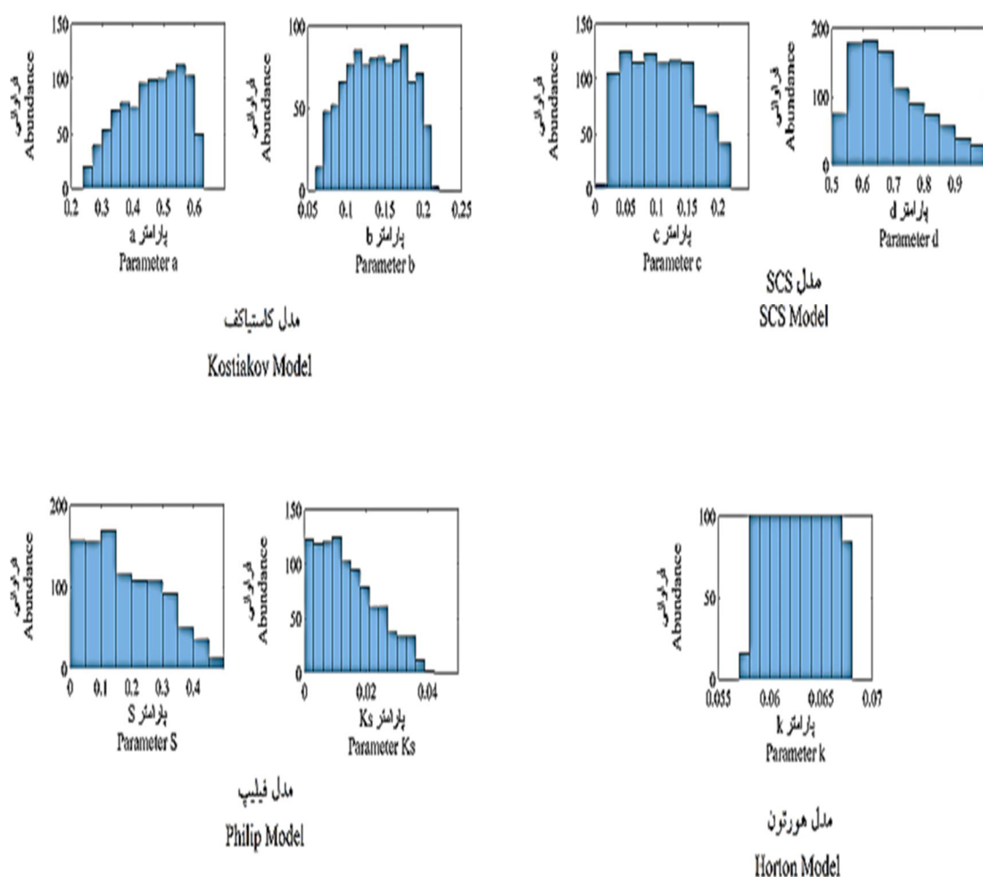
شکل ۳- توزیع‌های پسین مدل‌های نفوذ در خاک لوم رسی.
