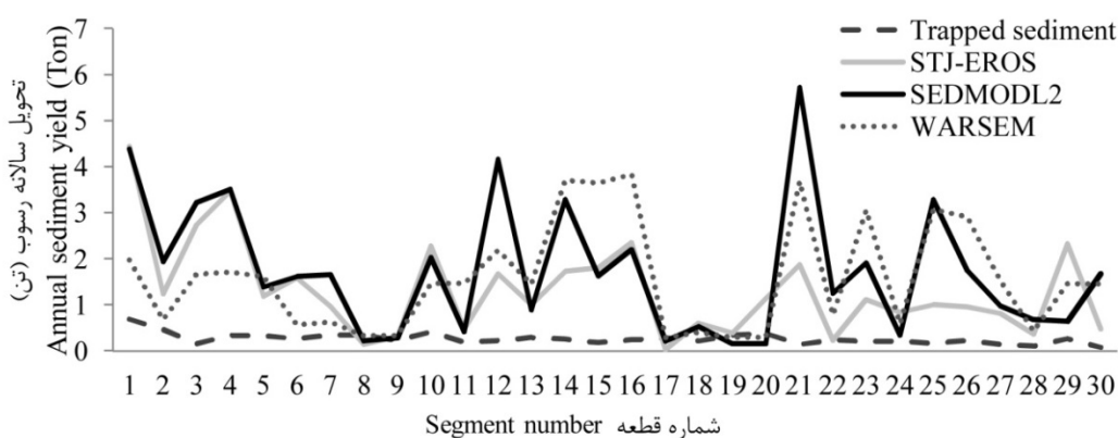
شکل ۵- مقدار تحویل سالانه رسوب قطعات مختلف جاده.
