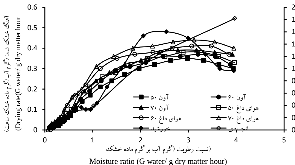
شکل ۳- تغییرات آهنگ خشک شدن نسبت به محتوی رطوبت برای روش های مختلف خشک کردن
