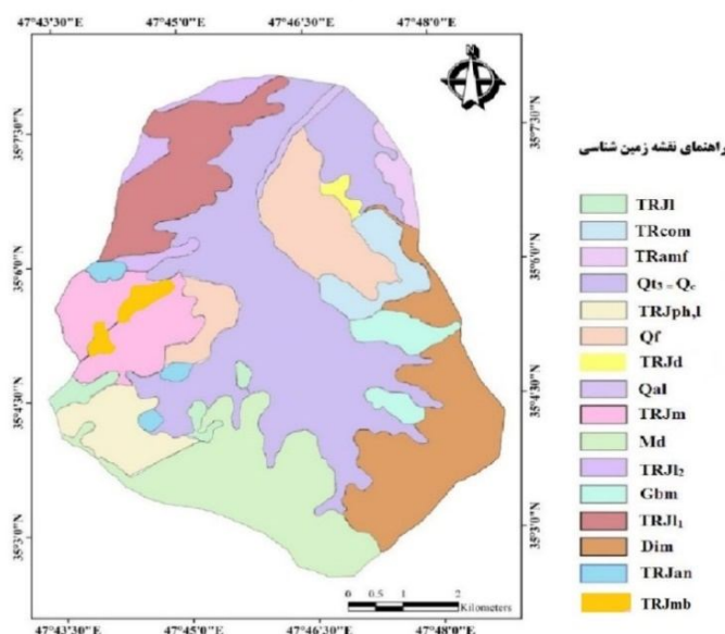
شکل ۲- زمین‌شناسی حوزه آبخیز بدر شهرستان قروه، استان کردستان. Figure 2. Geology of Badr watershed, Qorveh city, Kurdistan province.
