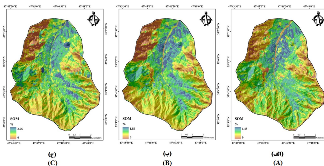
شکل ۴- نقشه‌های پیش‌بینی کربن آلی خاک با استفاده از رگرسیون خطی چندگانه. نقشه ب، پیش‌بینی مقدار میانگین، نقشه الف، پیش‌بینی با دامنه پراکندگی ۵ درصد کمتر از میانگین و نقشه ج، پیش‌بینی با دامنه پراکندگی ۵ درصد بیشتر از میانگین را نشان می‌دهند.
