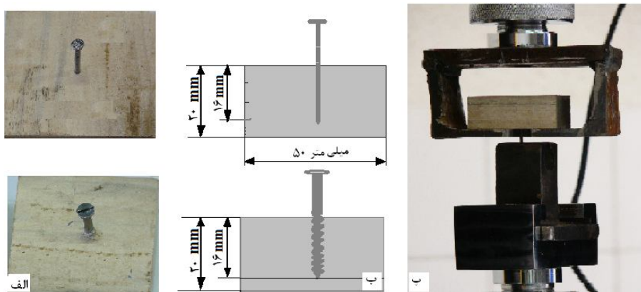
شکل ۲- الف) نمونه آزمونی، ب) شکل شماتیک نمونه‌ها حاوی اتصال دهنده‌ها و ب) چگونگی اندازه‌گیری قدرت نگهداری اتصال دهنده‌ها.
