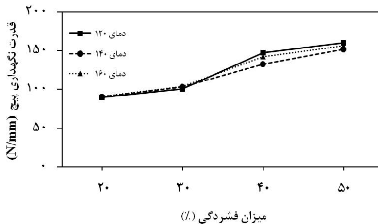
شکل ۵ - روند تغییرات قدرت نگهداری پیچ در چوب فشرده شده صنوبر.
