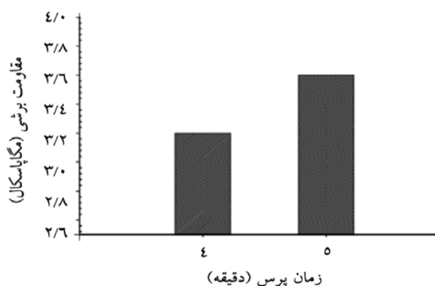
شکل ۴- اثر زمان پرس بر مقاومت برشی.
