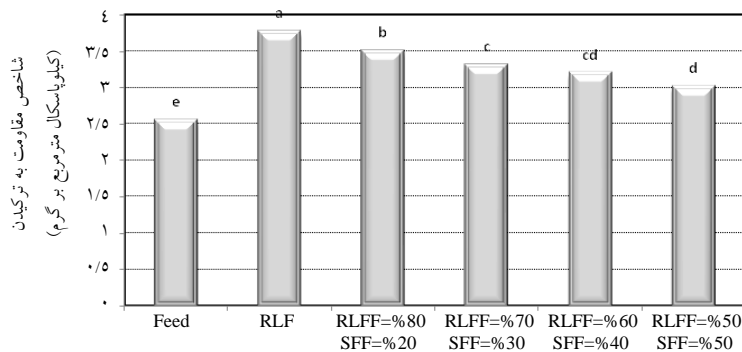
شکل ۱- گروه‌بندی دانکن مقادیر میانگین شاخص مقاومت به تراکدن کاغذهای دست‌ساز.
