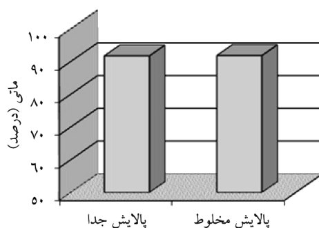
شکل ۱۵- مقایسه میانگین ماتی کاغذهای دست‌ساز به‌دست آمده از پالایش جداگانه و مخلوط خمیرهای CMP ممرز و الیاف بلند وارداتی.
