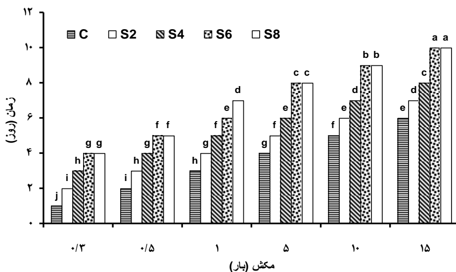
شکل ۳- زمان لازم برای رسیدن به مکش‌های مختلف در خاک شنی لوم با سطوح مختلف ابرجاذب استاکوزرب (مقایسه میانگین با استفاده از آزمون دانکن در سطح پنج درصد انجام شده است).
