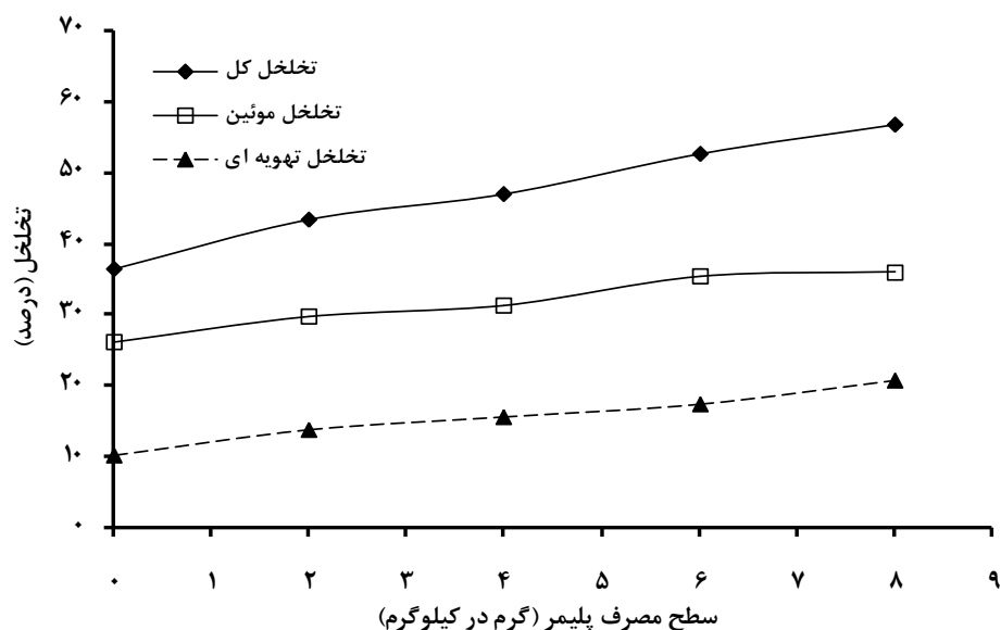
شکل ۹- مقایسه تخلخل کل، موئینی و تهویه‌ای خاک در بافت لوم شنی با سطوح مختلف پلیمر استاکوزرب.
