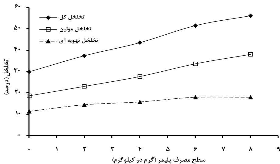
شکل ۶- مقایسه تخلخل کل، موئینی و تهویه‌ای خاک در بافت شنی لوم با سطوح مختلف پلیمر تراوات.
