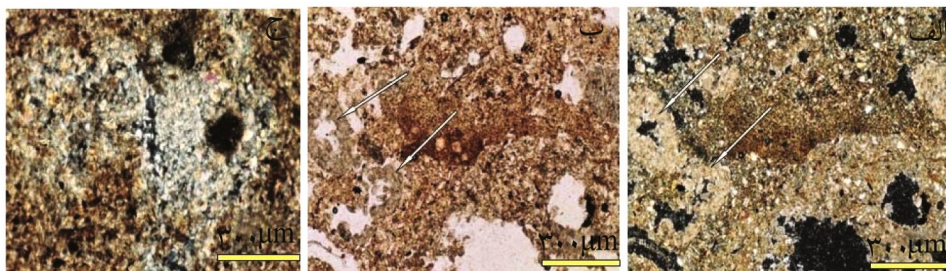
شکل ۱۰- الف و ب: کلسیت سیتومورفیک افق Bk خاک‌رخ ۵ الف: نور معمولی (PPL). ب: نور متقاطع (XPL). ج: پرشدگی به وسیله گچ افق C ۱ خاک‌رخ ۷ نور متقاطع (XPL).
