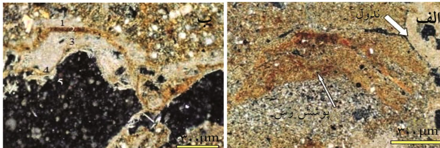
شکل ۸- الف: پوشش رس و ندول کلسیت افق Bk نور معمولی (PPL).
