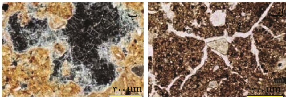
شکل ۹- الف: حفره نوع کانال و میکروساختمان مکعبی زاویه دار افق A خاکرخ ۲.
