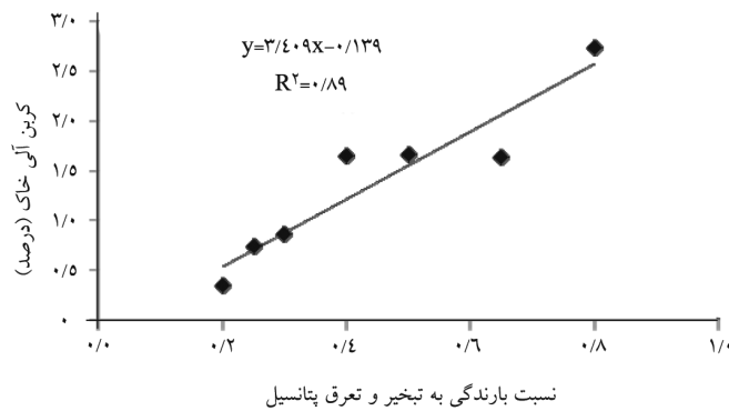
شکل ۳- رابطه کربن آلی خاک و شاخص اقلیمی در منطقه مورد مطالعه.
