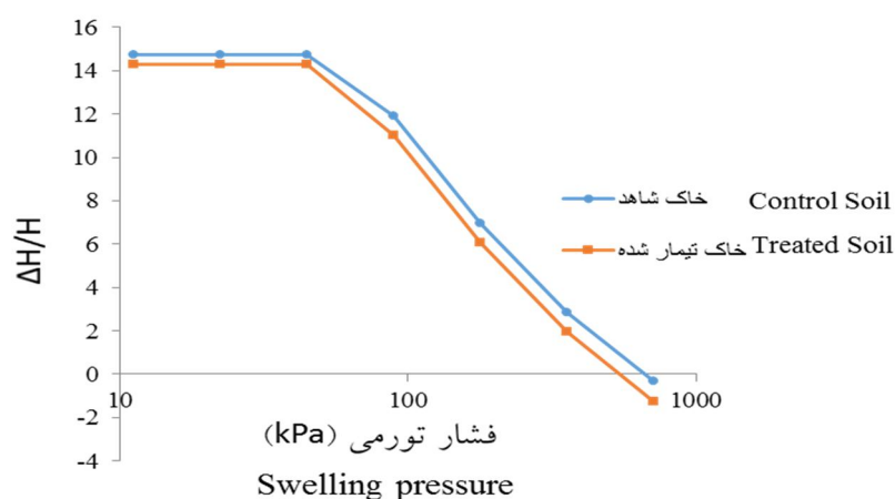
شکل ۵- نمودار حاصل از آزمایش فشار تورمی خاک تیمار شده و شاهد. Figure 5. Swelling pressure test plot of treated and control soil.
