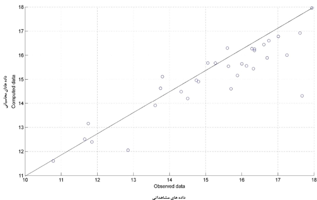
شکل ۵- مقایسه نتایج داده‌های مشاهده‌ای و محاسباتی در دوره صحت‌سنجی (m) برای چاه چگنی.
