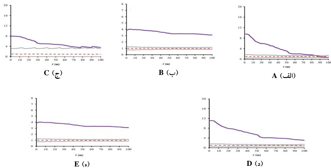
شکل ۴- تابع g(r) نشان‌دهنده پراکنش مکانی: اراضی مسطح (الف)، جهت شمالی (ب)، جهت شرقی (ج)، جهت جنوبی (د) و جهت غربی (ه)، در محدوده مورد مطالعه. خط بنفش بیانگر تغییرات مشاهده شده و خطوط خاکستری محدوده شبیه‌سازی شده با ۱۹۹ بار تکرار آزمون مونت کارلو و خط چین نشان‌دهنده حالت پیش فرض است.
