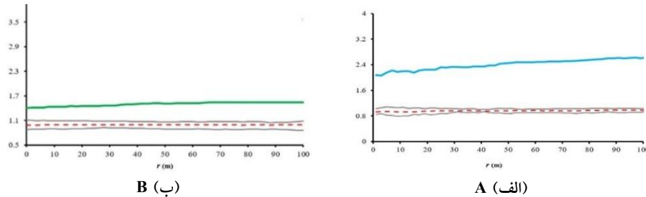
شکل ۷- ارتباط متقابل تراکم آبراهه‌ها و دامنه‌های شمالی: براساس تابع g_{12}(r) ، خط آبی بیانگر تغییرات مشاهده شده (الف) و براساس تابع O\text{-ring}_{12}(r) ، خط سبز بیانگر تغییرات مشاهده شده (ب). خطوط خاکستری محدوده شبیه‌سازی شده با ۱۹۹ بار تکرار آزمون مونت‌کارلو و خط چین قرمز نشان‌دهنده حالت پیش‌فرض است.
