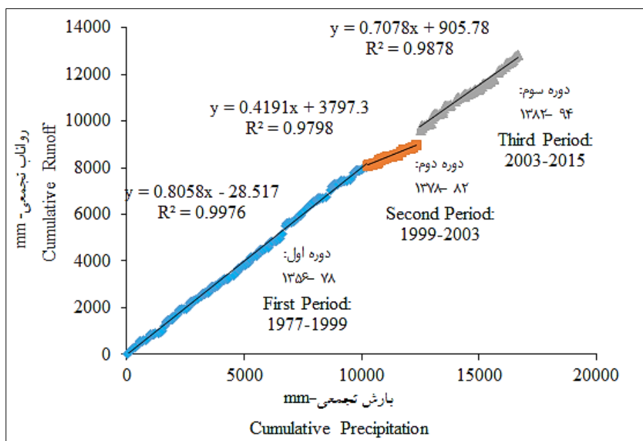
شکل ۲- منحنی جرم مضاعف بارش- رواناب، حوزه آبخیز کند.
