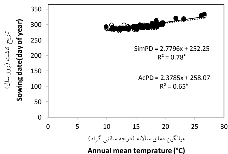
شکل ۳- رابطه بین تاریخ کاشت و میانگین دمای روزانه در مکان‌های زیر کشت جو آبی. مقادیر تاریخ کاشت واقعی (AcPD) و تاریخ کاشت شبیه‌سازی شده (SimPD) مورد بررسی قرار گرفتند. (●): تاریخ کاشت واقعی، ○: تاریخ کاشت شبیه‌سازی شده، خط پیوسته: رگرسیون بین تاریخ‌های کاشت شبیه‌سازی شده، نقطه‌چین: رگرسیون بین تاریخ‌های کاشت واقعی).
